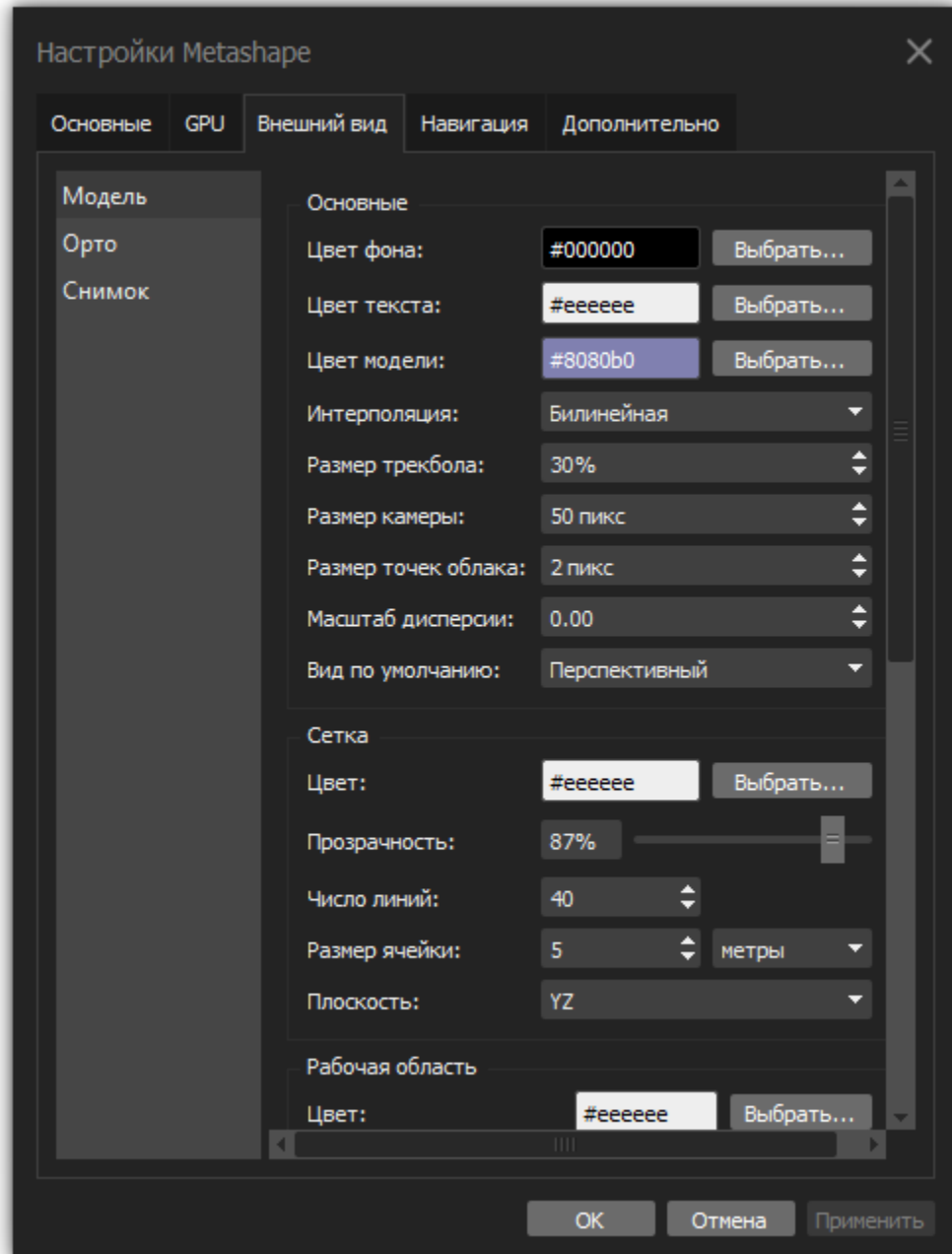
Вкладка Внешний вид (Режим просмотра Модель)
